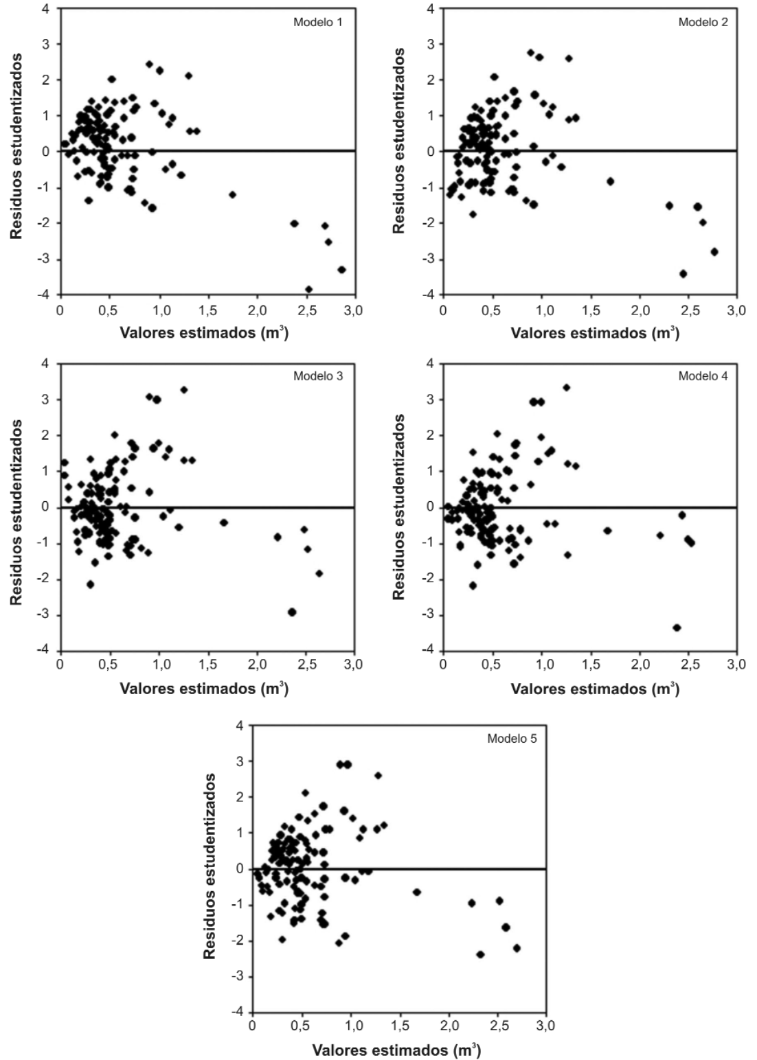
Figura 1. Relación entre los residuos estudentizados y valores estimados de volumen total ( m^3 ) a partir de las ecuaciones de volumen ajustadas.
