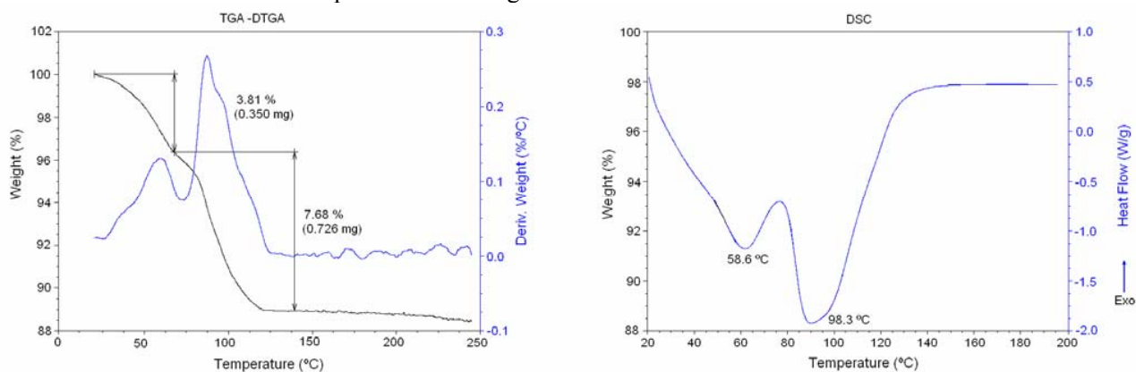
Figura 1. Curvas TGA-DTGA y DSC para el complejo K_3Fe(C_2O_4)_3 \cdot 3H_2O .
