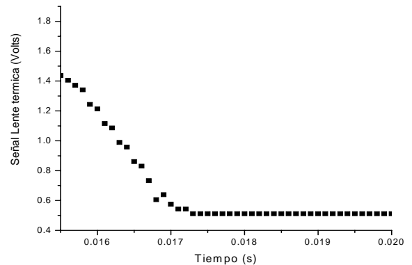
Figura 5. Curva experimental de la respuesta de la lente térmica, para una muestra de aceite de oliva
