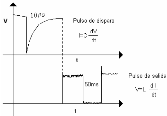
Figura 4. Diagrama de tiempos de la entrada y la salida del pulso De 10 \mu s y 50 ms, respectivamente.
