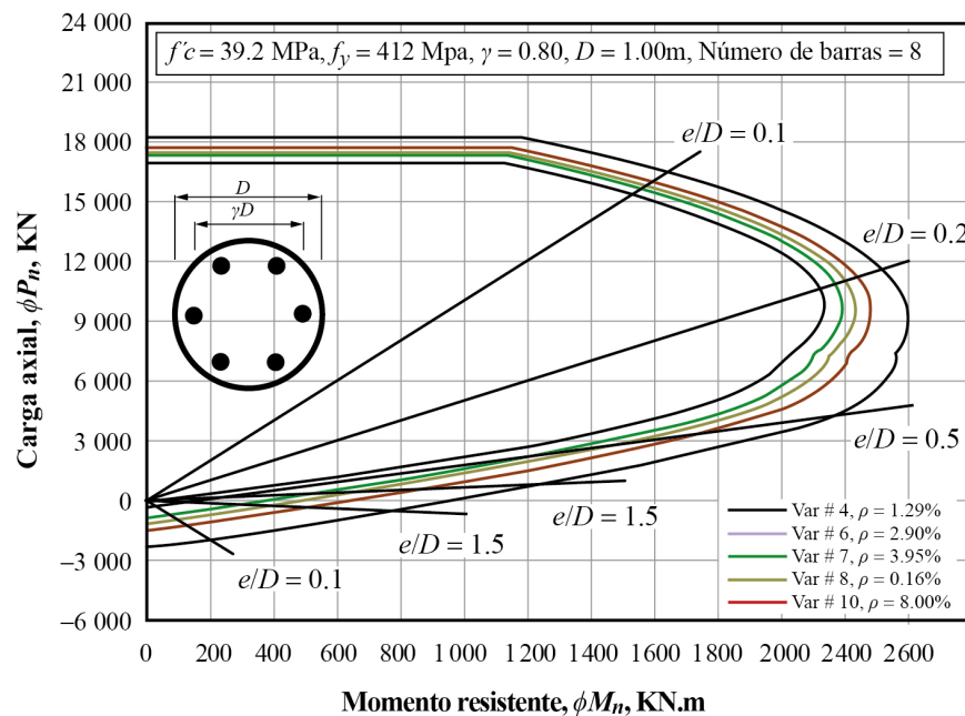
GRÁFICA 14 Diagrama resistente de interacción con 8 barras de refuerzo Diagrama de interacción c39.2-412.80-1.00-8 Fuente: elaboración propia.
