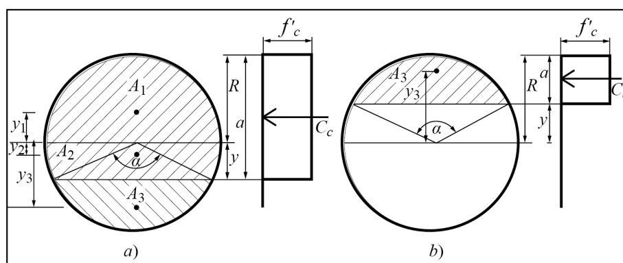
FIGURA 3 Condiciones de la profundidad del bloque de esfuerzos Fuente: elaboración propia. Nota: a) a \geq R ; b) a < R .
