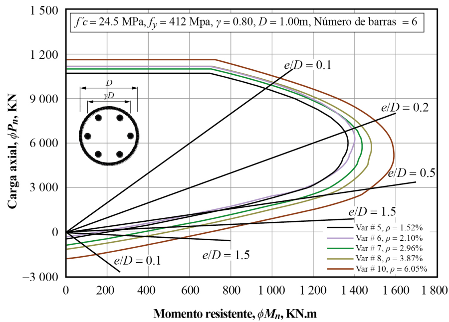
GRÁFICA 13 Diagrama resistente de interacción con 6 barras de refuerzo Diagrama de interacción c24.5-412.80-1.00-6 Fuente: elaboración propia.
