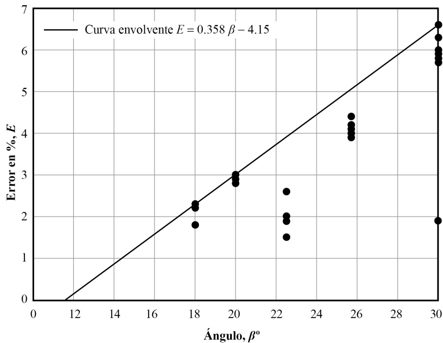
GRÁFICA 12 Relación ángulo \beta -error ( E )
