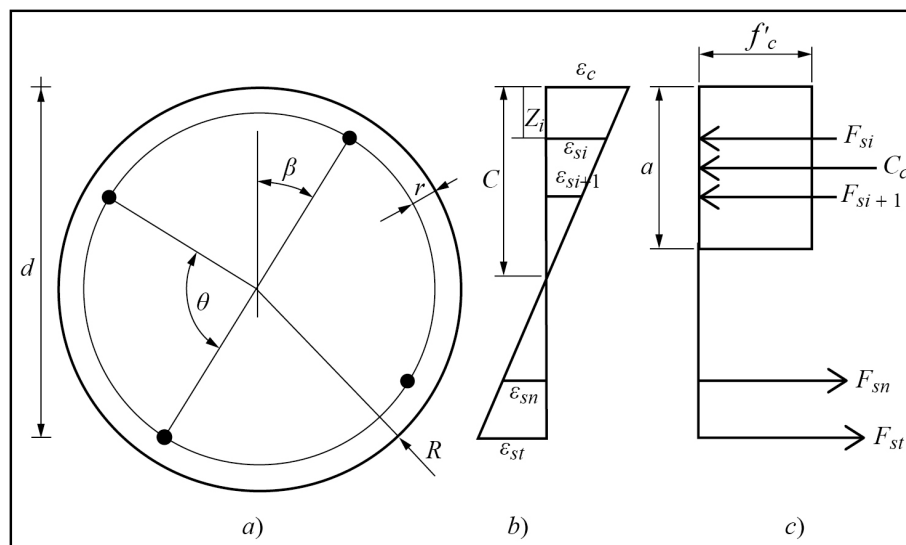
FIGURA 2 Geometría de una columna sólida
