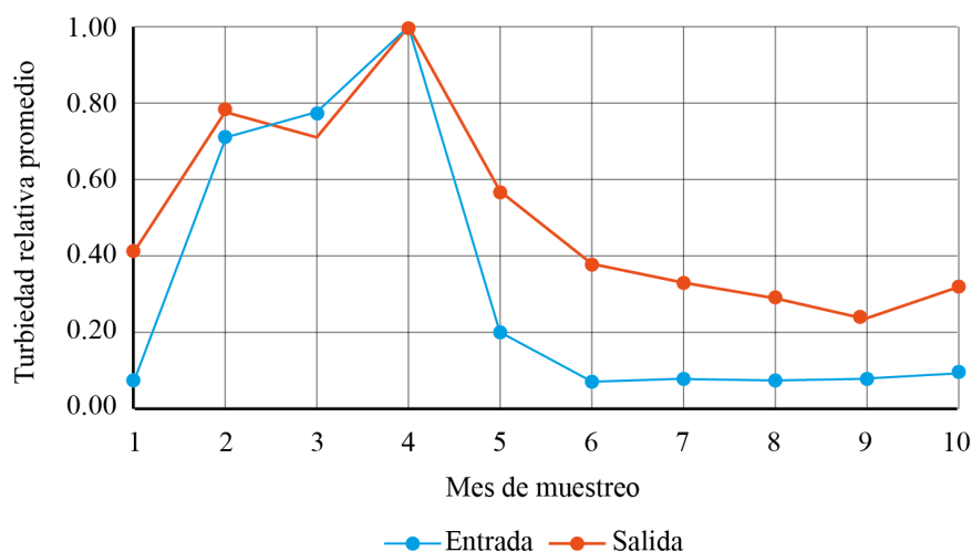
GRÁFICA 1 Variación relativa de la turbiedad promedio a la entrada y salida de la planta
