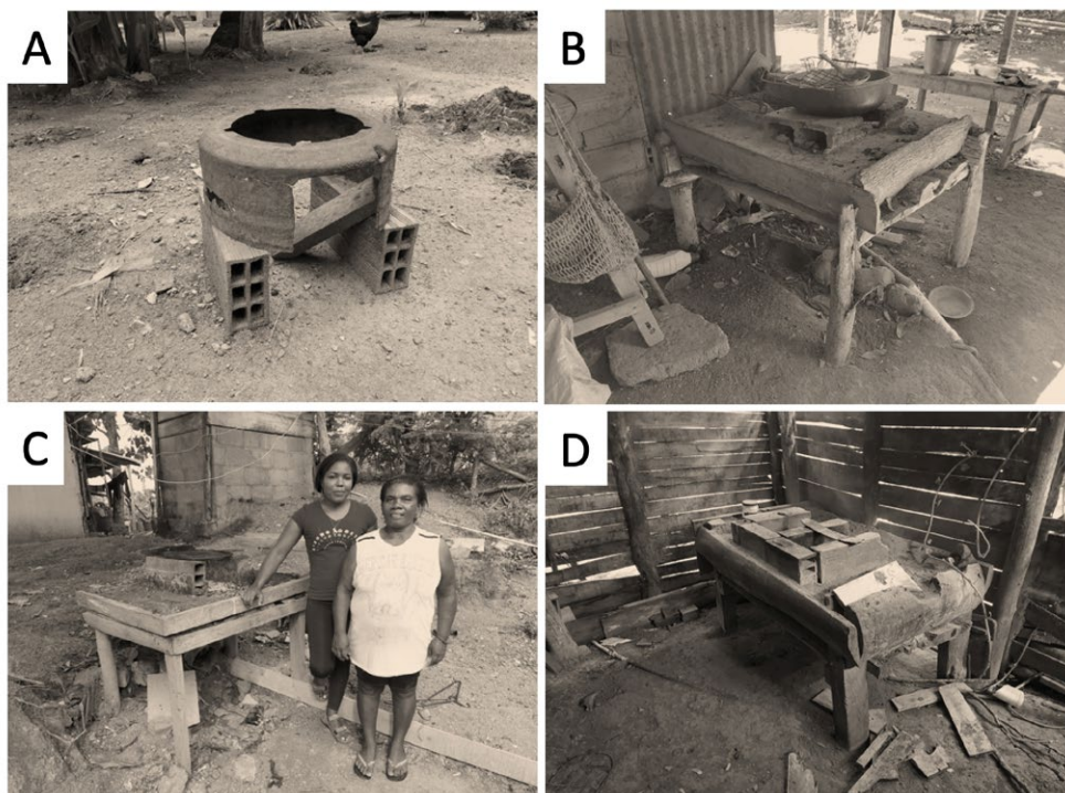
Figura 9. Tipología de fogones en el municipio de Necoclí. (A) Binde metálico; (B) (C) (D) Fogones de banco con estructura en madera.
