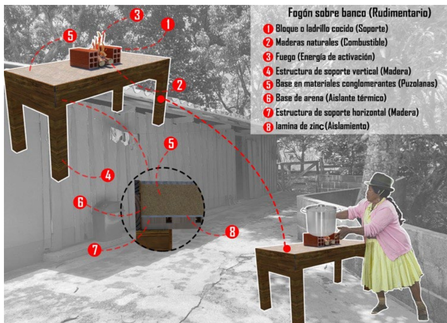
Figura 5. Componentes del fogón de banco con estructura en madera.
