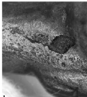
Figura 10 – Detalle de la falta de metal en las piernas de la estatuilla femenina en plata ME I 281 elaborada por vaciado
