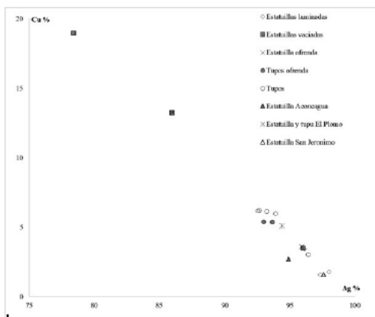
Figura 12 – Comparación de las concentraciones de plata (Ag %) y cobre (Cu %) determinadas por FRX para los tupus y las estatuillas del hallazgo de Paucartambo y valores publicados para las estatuillas y tupus de San Jerónimo (Rovira Llórens y Gómez Ramos, 1995), Cerro Aconcagua (Bárcena, 2004) y Cerro El Plomo (Oberhauser et al., 1059). Elaborado por J. C. S. Palminos & M. F. Guerra
