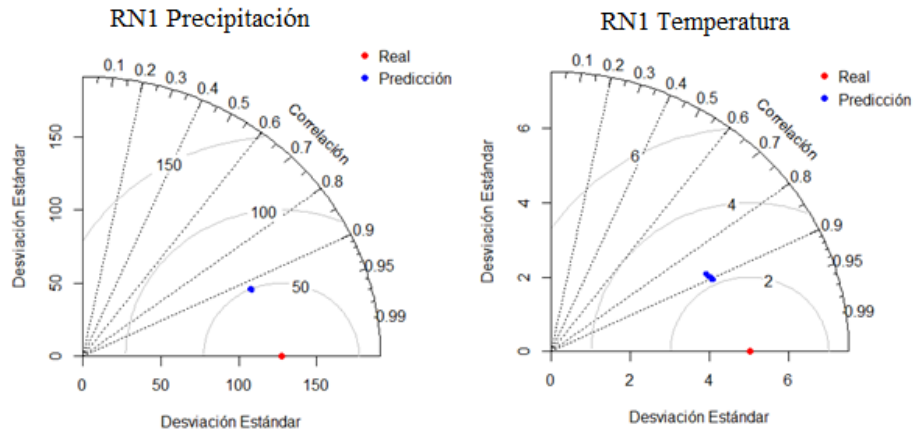
Figura 12 Diagrama de Taylor de RN1 para precipitación y temperatura. Elaboración Propia.
