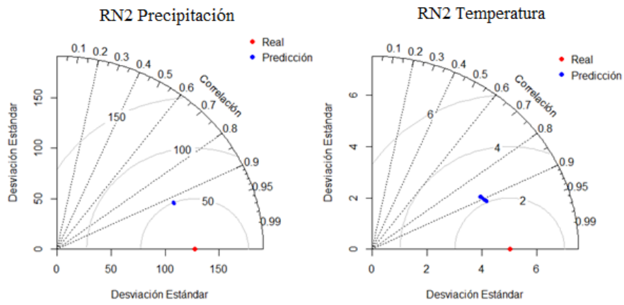
Figura 13 Diagrama de Taylor de RN2 para precipitación y temperatura. Elaboración Propia
