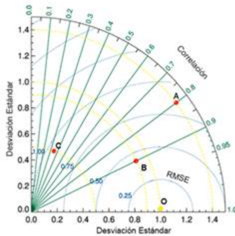
Figura 8. Diagrama de Taylor. Elaboración Propia.
