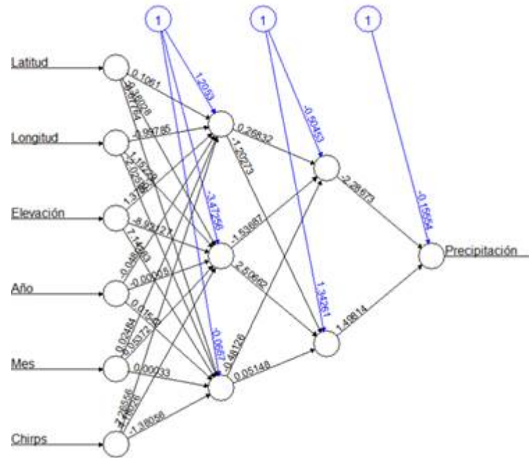
Figura 9 Red neuronal artificial para precipitación usando la topología 6-3-2-1. Elaboración Propia
