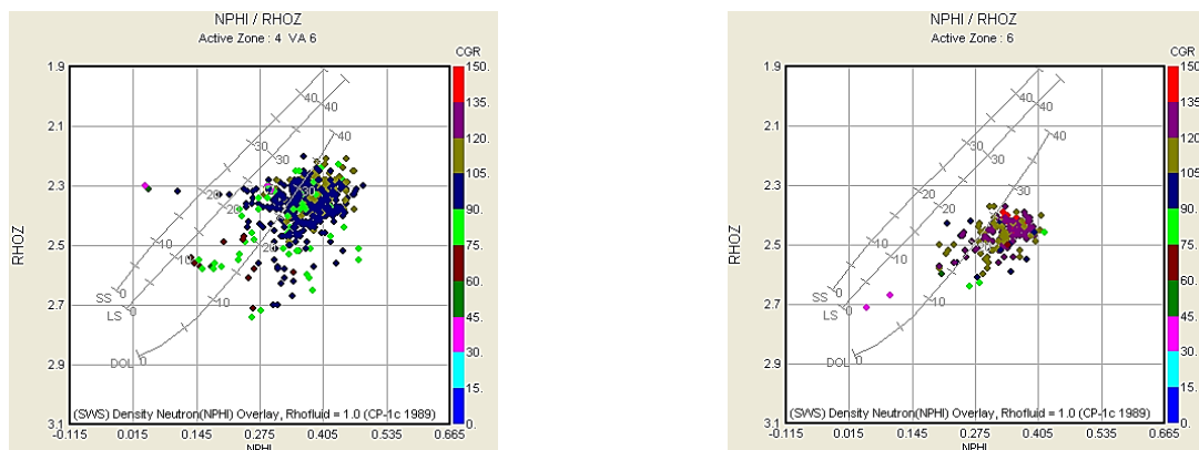
Figura 12. Gráfico de propiedades cruzadas de los pozos YUM-211RE (izquierda) y YUM-400 (derecha)
