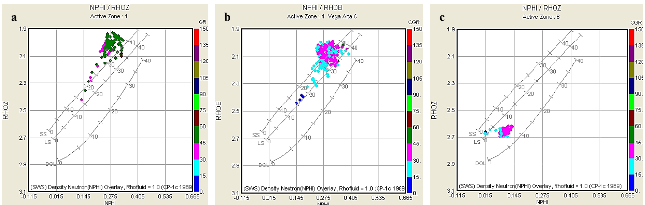
Figura 9. Gráfico de propiedades cruzadas de los pozos FRN-1002ST (a), STC-100 (b) y YUM-400 (c), con grupos de puntos que indican homogeneidad por su arenía.
