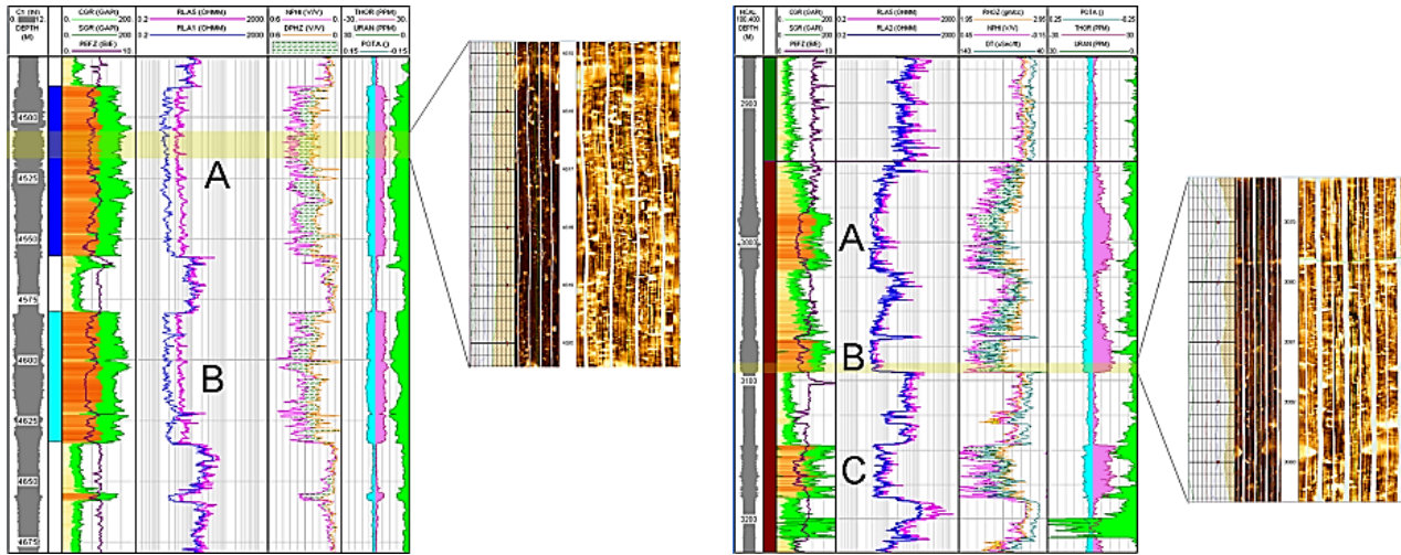
Figura 13. Izquierda: Registro compuesto del pozo YUM 211-RE2 con los intervalos arcillosos A y B; A representado en la imagen de FMI. Derecha: pozo YUM-400 con los intervalos arcillosos A, B y C; B en la imagen.
