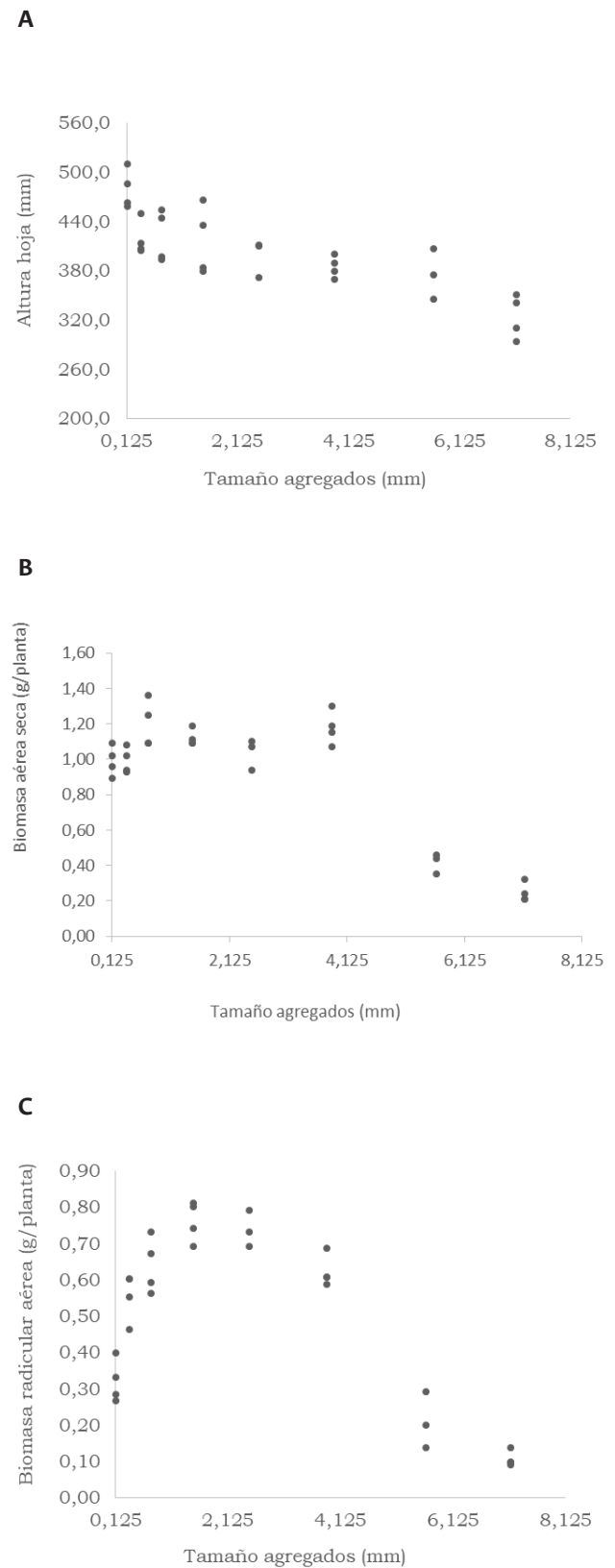
Figura 2. Altura (A) y biomasa seca aérea (B) y radical seca (C) de pasto guinea ( Megathyrsus maximus cv. Mombasa) en función del tamaño medio de agregados de un Inceptisol de bosque seco tropical de Colombia.
