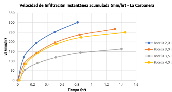
Figura 3. Comportamiento de la vii (mm/hr) para los goteros en La Carbonera, Pradera.
