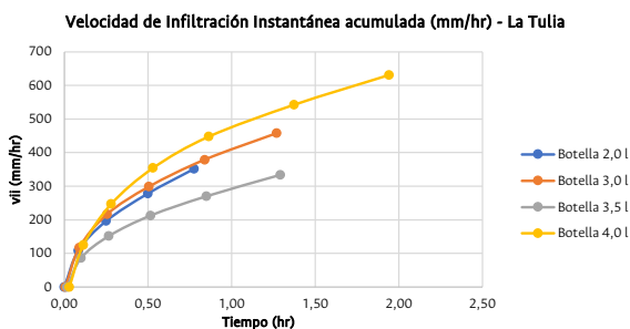
Figura 4. Comportamiento de la vii (mm/hr) para los goteros en Villa Hermosa, Dagua.
