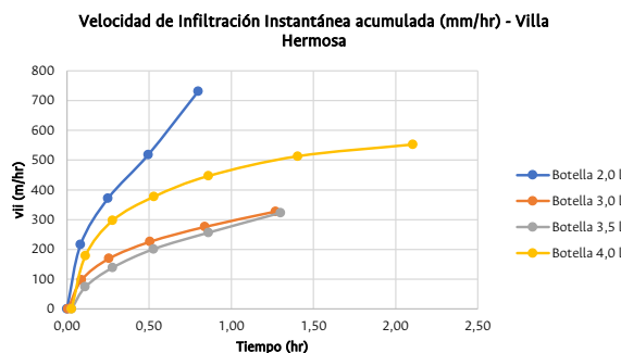
Figura 4. Comportamiento de la vii (mm/hr) para los goteros en Villa Hermosa, Dagua.
