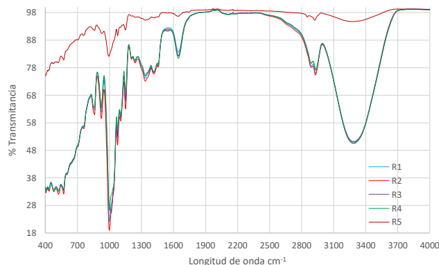
Figura 4. FTIR de las películas fabricadas.
