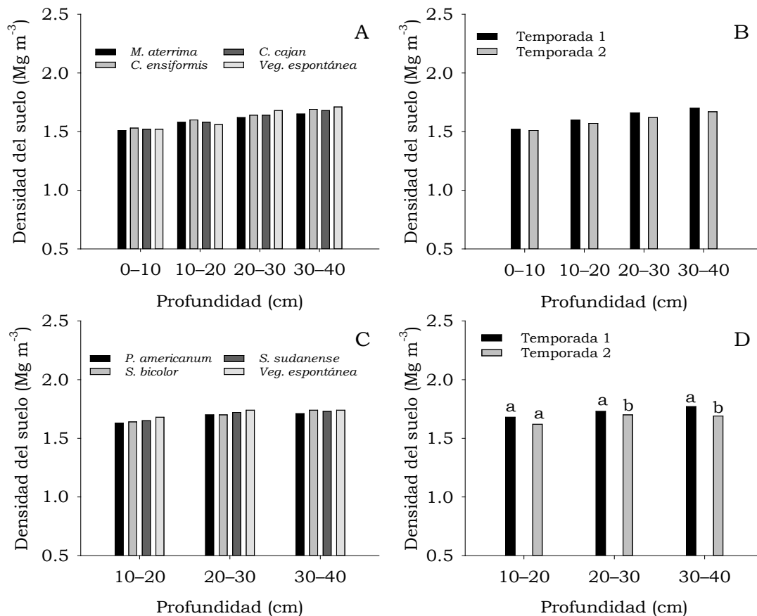
Figura 3. Densidad del suelo a profundidades de 0-10, 10-20, 20-30 y 30-40 cm antes y después del cultivo de leguminosas (A y B) y gramíneas (C y D). Medias seguidas de letras minúsculas iguales en la columna no difieren entre sí por la prueba de Tukey ( p < 0,05 ). Fuente: elaboración propia.
