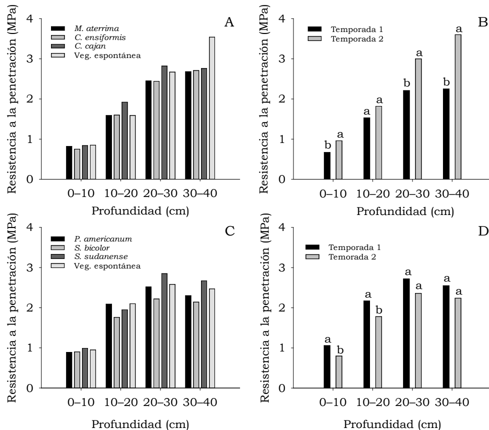
Figura 5. Resistencia a la penetración a profundidades de 0-10, 10-20, 20-30 y 30-40 cm antes y después del cultivo de leguminosas (A y B) y gramíneas (C y D). Medias seguidas de letras minúsculas iguales en la columna no difieren entre sí por la prueba de Tukey ( p < 0.05 ). Fuente: elaboración propia.
