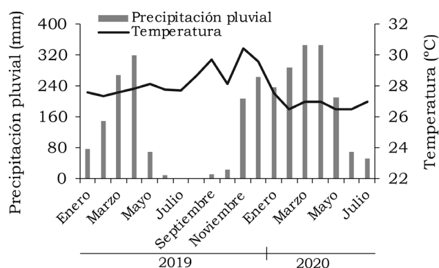
Figura 1. Precipitación y temperatura del aire en el municipio de Chapadinha-MA, Brasil, durante el desarrollo del experimento. Fuente: INMET, 2020. .
