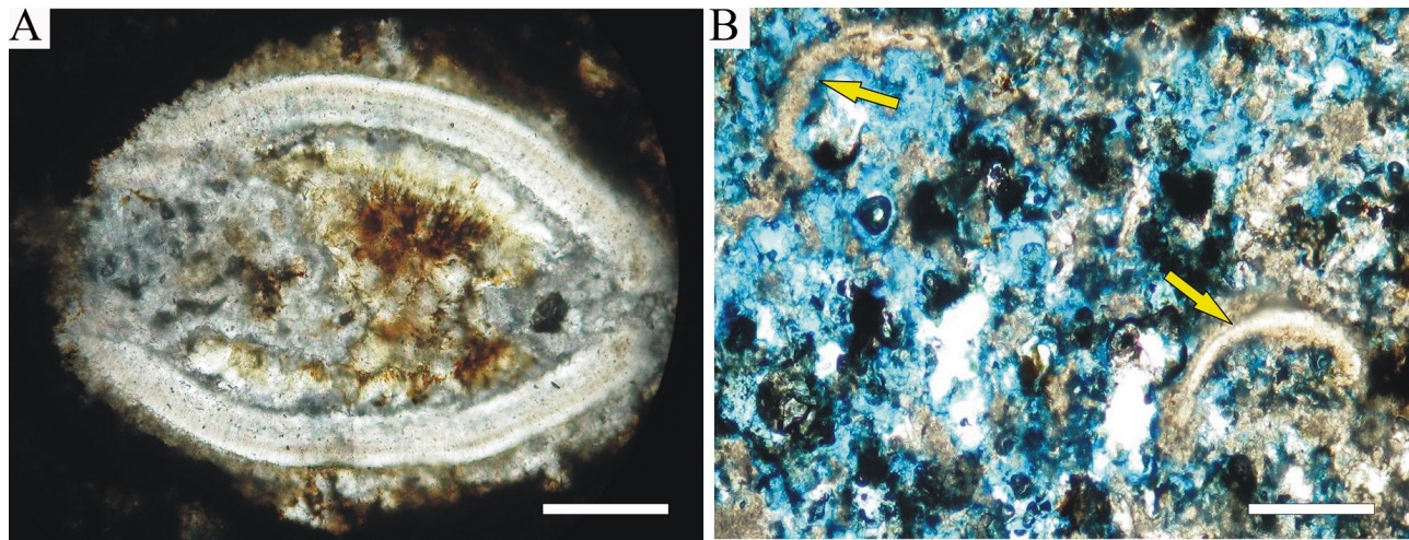
FIG. 5. Restos de probables ostrácodos observados en microscopio petrográfico a nicos cruzados en E1. A. Valvas articuladas, escala: 0,25mm. B. Valvas desarticuladas no fragmentadas, escala: 0,5 mm.
