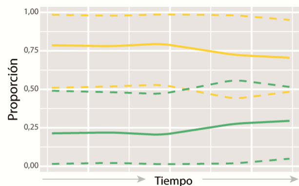
B326 ( M_2 )
