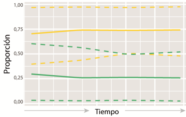
B776 ( M_1 )
