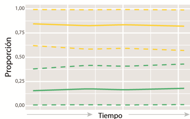
B409 ( M^3 )
