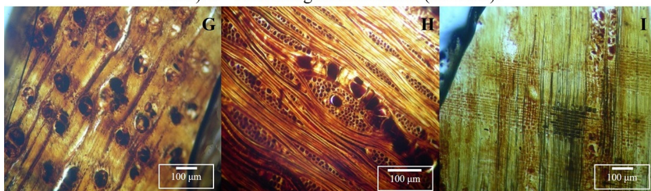
Schinopsis sp. G- Vista Transversal (ID 6581). H- Vista Longitudinal Tangencial (ID 7144). I- Vista Longitudinal Radial (ID 6580).
