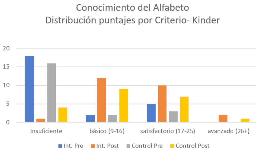
Figura 1. Resultados Conocimiento del Alfabeto Kinder
