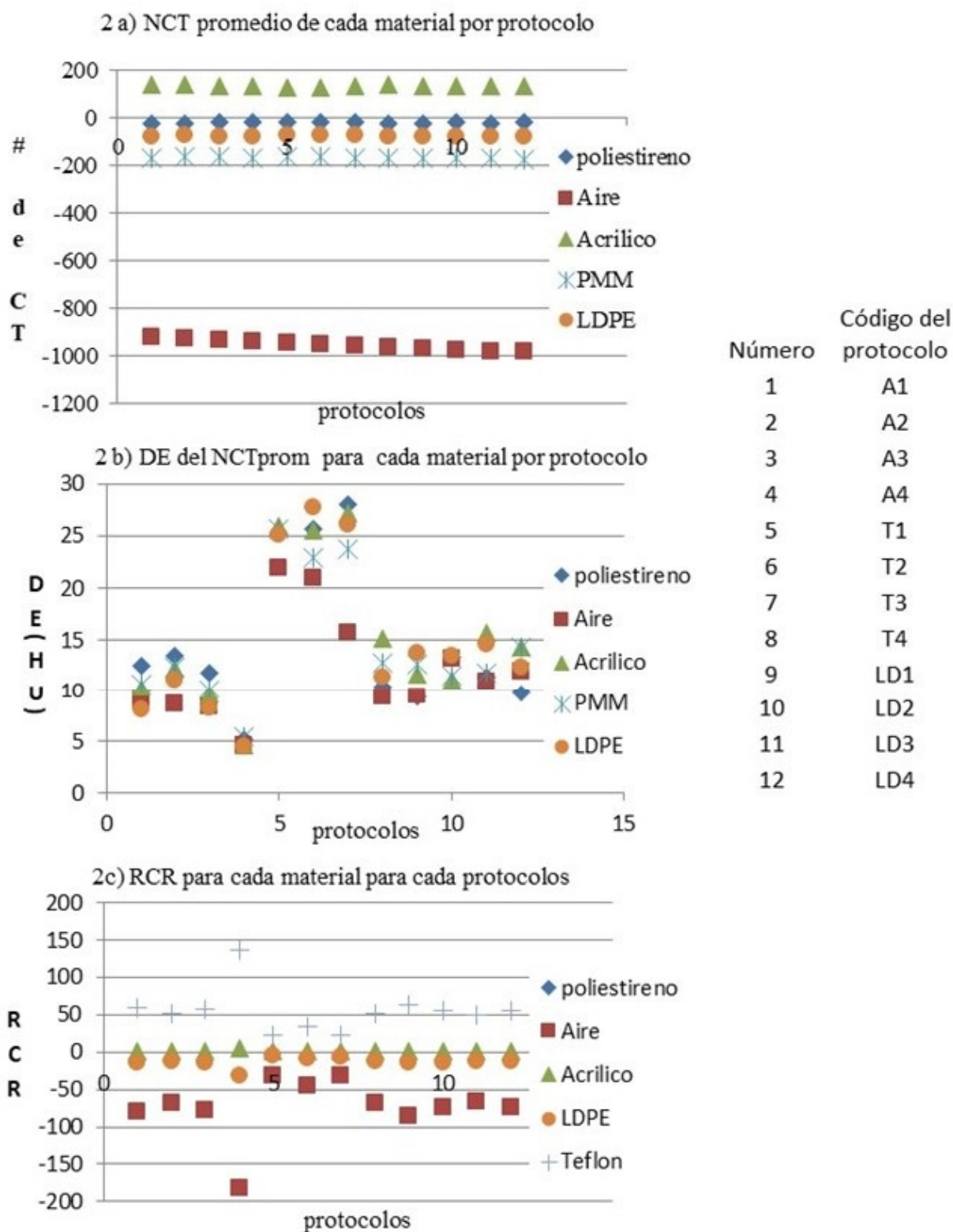
Fig. 2. Gráficos que muestran los resultados del a) número de Hounsfield promedio por material para cada protocolo, b) desviación estándar del NCT para cada protocolo, c) Relación contraste ruido para cada material
