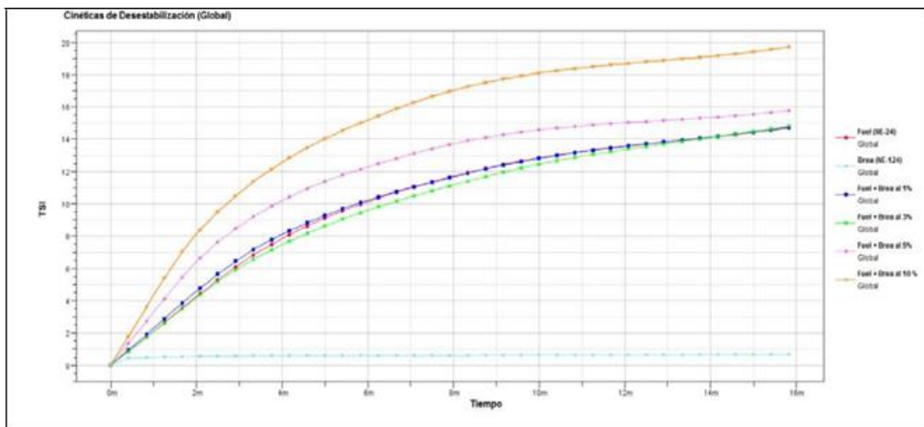
Fig. 7. Comportamiento del TSI en los 15 minutos de prueba de fuel oil, residuo de brea y sus mezclas.
