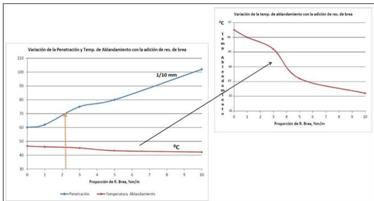
Fig. 3. Gráfica representativa del comportamiento de la penetración y temperatura de ablandamiento en las mezclas cemento asfáltico- residuo de brea de hulla.
