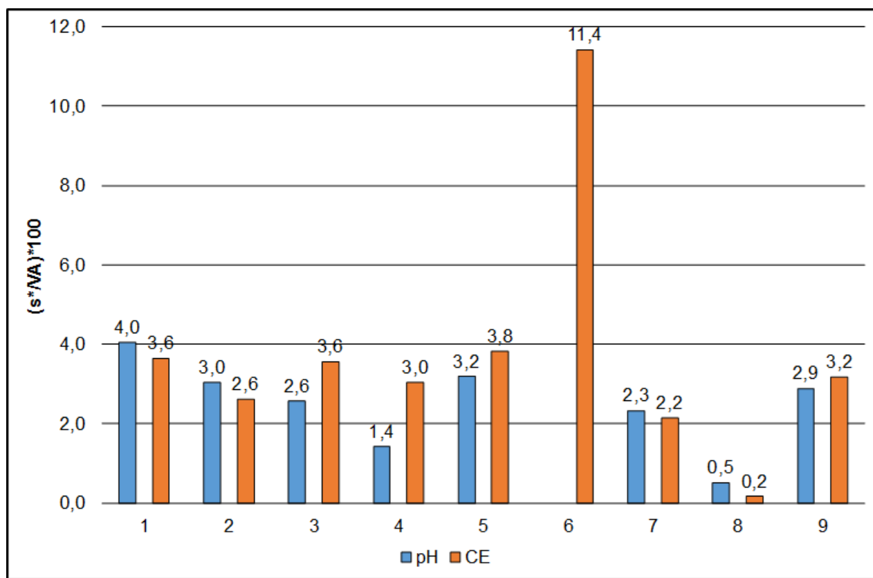
Fig. 3. Comportamiento del Coeficiente de Variación (CV) calculado a partir del Valor Asignado (VA) y de s^* (Desviación estándar para la evaluación de la aptitud), en los diferentes EA para el pH y la CE.
