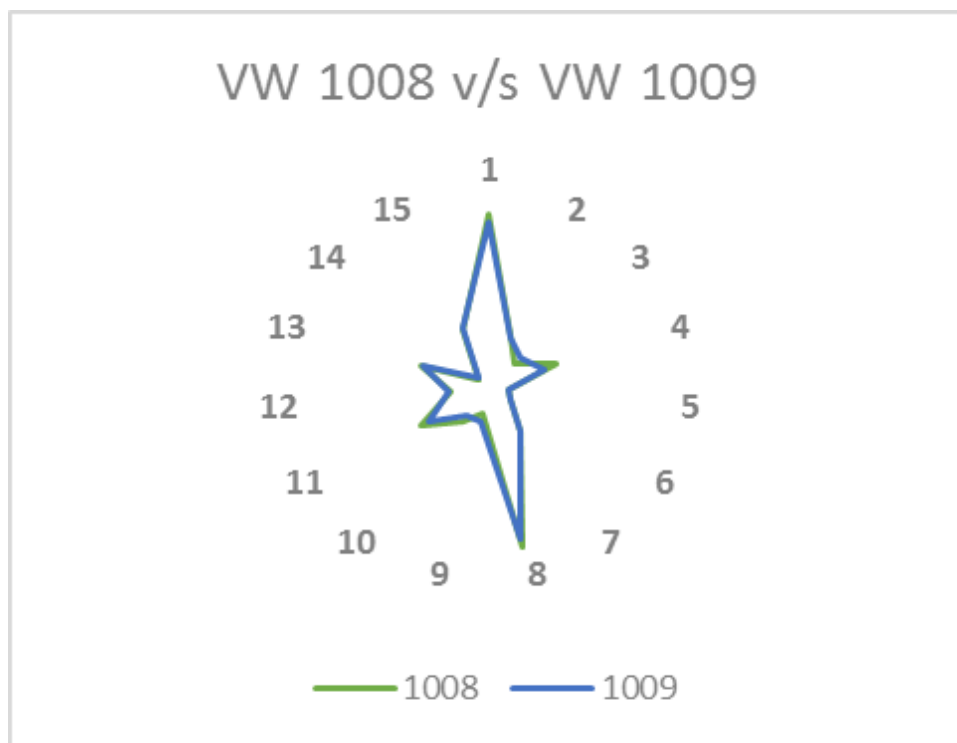
Fig. 8. Diagrama de estrella de la comparación de los pozos VW 1008 y 1009, mostrando problemas de comunicación entre ellos (diferencia de 9.42%).
