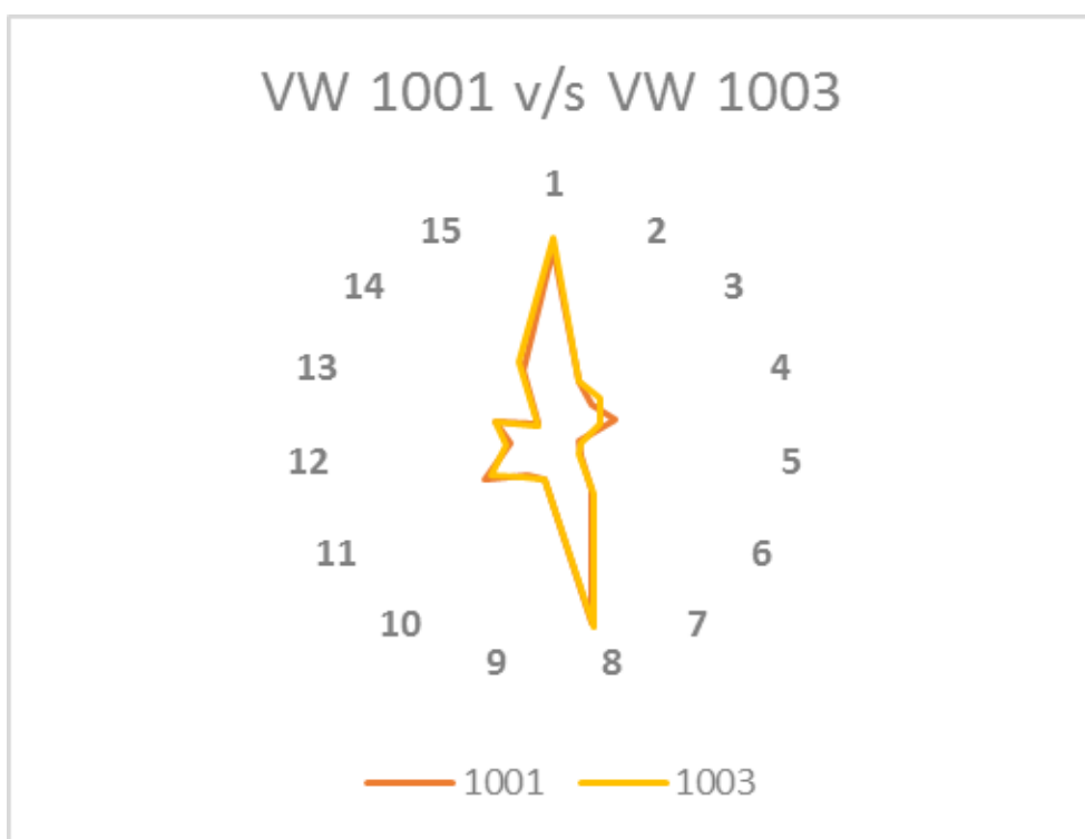
Fig. 6. Diagrama de estrella de la comparación de los pozos VW 1001 y 1003, mostrando problemas de comunicación entre ellos (diferencia de 8.44%).
