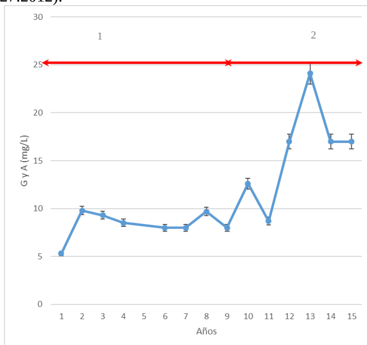
Fig. 7. Comportamiento de las grasas y aceites durante todo el período de estudio.
