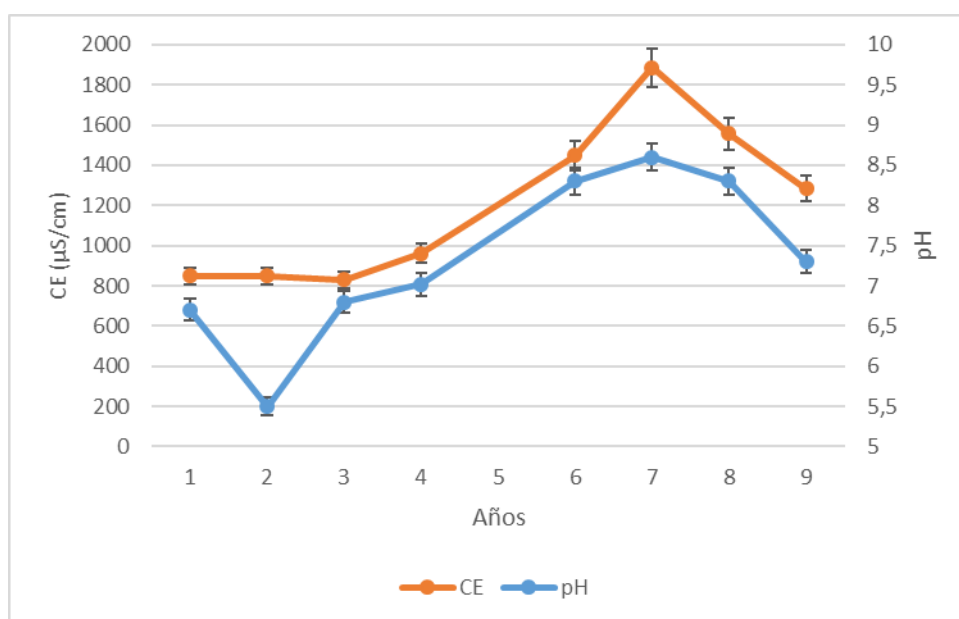
Fig. 4. Comportamiento del pH y la conductividad eléctrica (CE) durante los estudios previos de las aguas residuales generadas en la Empresa.
