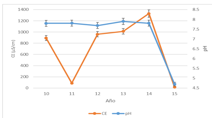
Fig. 6. Comportamiento del pH y la conductividad eléctrica (CE) después de la introducción de la planta de aceites ozonizados.
