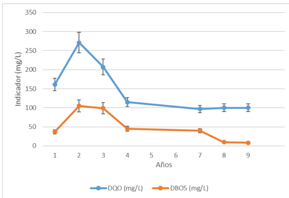
Fig. 3. Comportamiento de la DQO y DBO 5 de las aguas residuales generadas en la Empresa en los estudios previos.
