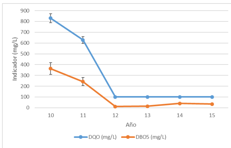
Fig. 5. Comportamiento de la DQO y DBO 5 de las aguas residuales vertidas en la Empresa CNIC después de la puesta en marcha de la planta de aceites ozonizados.
