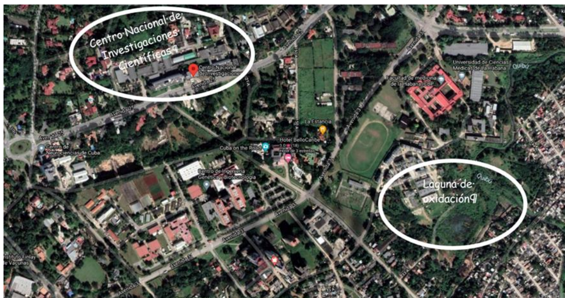
Fig. 2. Ubicación del área de estudio y el cuerpo receptor final de la zona.
