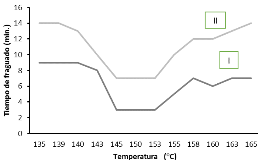
Fig. 2. Variación del tiempo de fraguado inicial (I) y final (II) del yeso especial, en el rango de temperatura.
