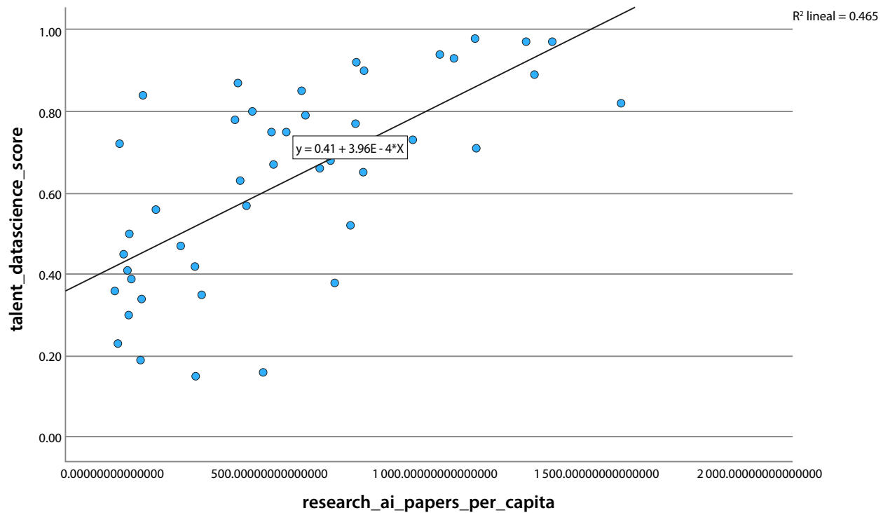
Figura 1. Relación entre publicaciones de inteligencia artificial per cápita y la puntuación de talento en ciencia de datos
