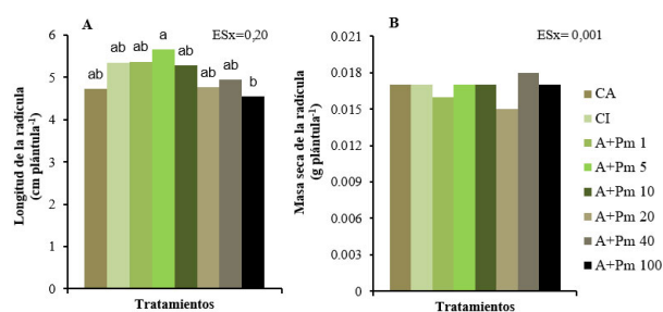
Figura 2. Efecto de Azofert®-F (A) y Pectimorf® (Pm) en la longitud (A) y en la masa seca de la radícula (B) de semillas de frijol Cuba Cueto-25-9-N, evaluadas a las 96 horas. CA: semillas sin tratar con los bioproductos, CI: semillas sólo tratadas con Azofert®-F. Pm 1-100: concentraciones de Pectimorf® en mg L -1
