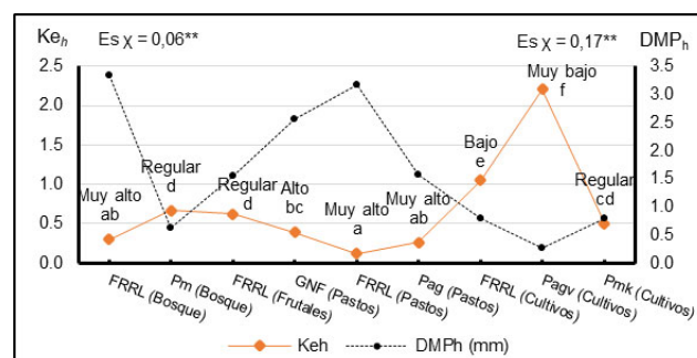
Figura 3. Calibración de los valores del coeficiente de estabilidad en húmedo ( Ke_h ) y su relación con el DMP_h en los diferentes tipos de suelos, según su uso. FRRL: Ferralítico Rojo Lixiviado, Pm: Pardo mullido GNF: Gley Nodular Ferruginoso, Pag: Pardo agrogénico, Pagv: Pardo agrogénico vértico, Pmk: Pardo mullido carbonatado
