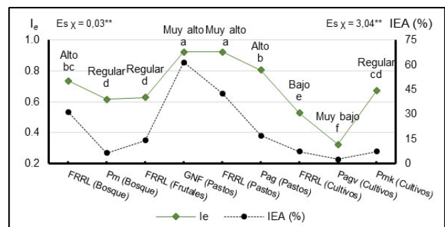
Figura 4. Calibración de los valores del Índice de estabilidad estructural ( I_e ) y su relación con el porcentaje del Índice de estabilidad de los agregados (IEA) determinado a partir del diámetro medio ponderado de los agregados en los diferentes tipos de suelos. FRRL: Ferralítico Rojo Lixiviado, Pm: Pardo mullido, GNF: Gley Nodular Ferruginoso, Pag: Pardo agrogénico, Pagv: Pardo agrogénico vértico, Pmk: Pardo mullido carbonatado
