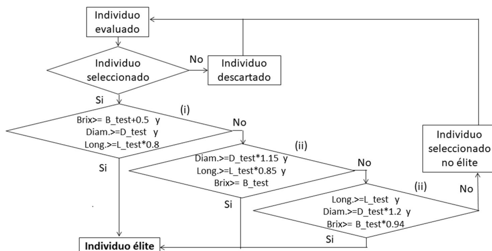
Figura 1. Algoritmo de detección de individuos élite en las etapas de propagación clonal 1 y 2
