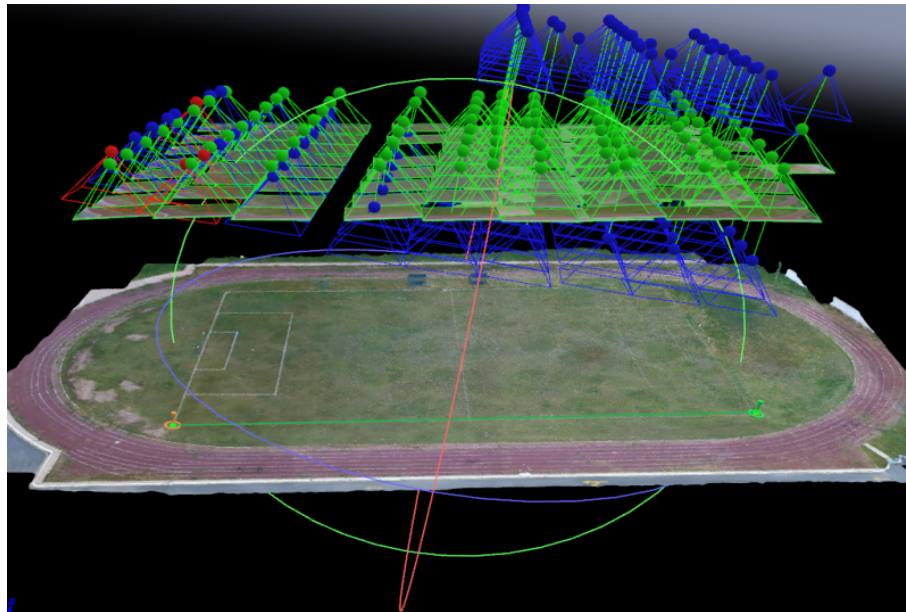
Fig.11 Ortomosaico del campo de futbol con 103 imágenes Elaborada por el autor.
