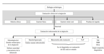
Algoritmo 1
