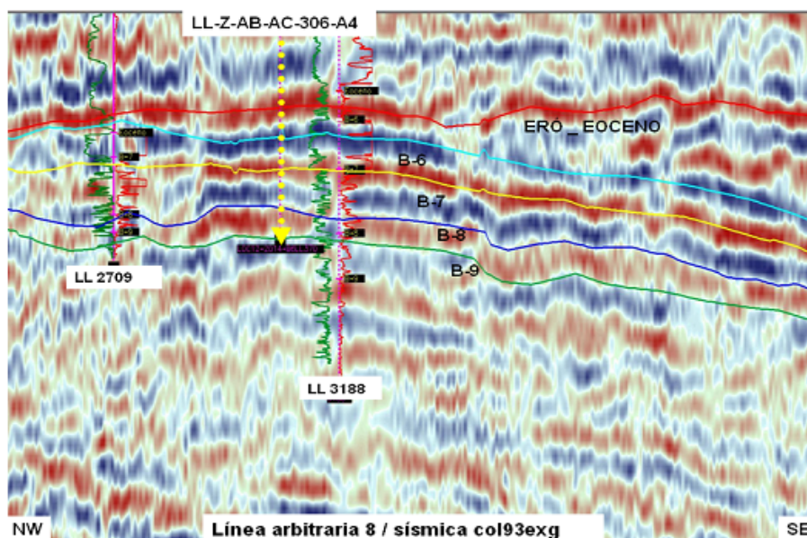
FIGURA 4. Línea sísmica de dirección NO-SE.
