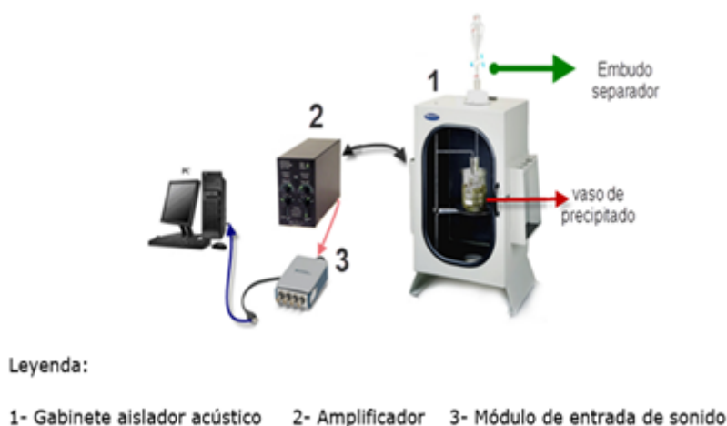
FIGURA 1. Instalación experimental de la técnica de emisión acústica.
