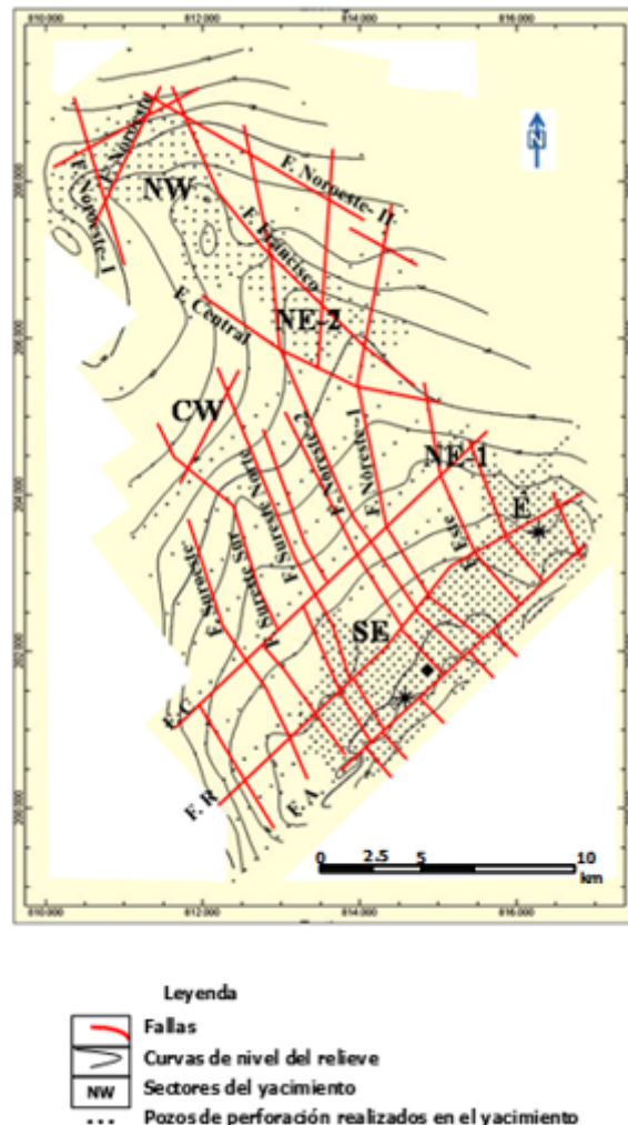
FIGURA 6. Interpretación estructural 2D del sistema de fallas y fracturas San Felipe determinado por la presente investigación.
