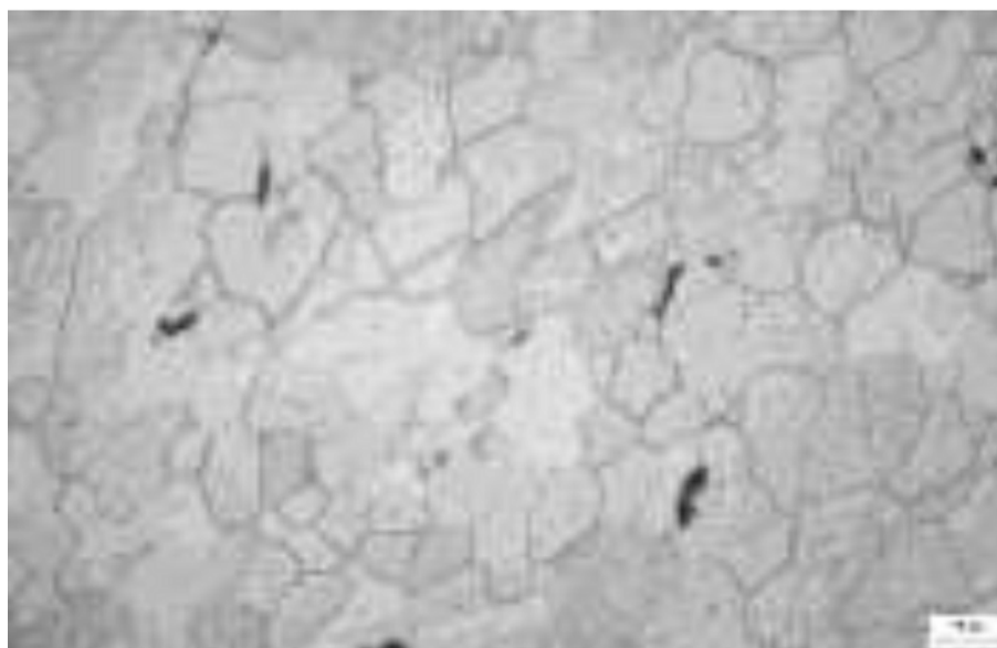
Fig. 4 Metalografía de acero AISI 1018
