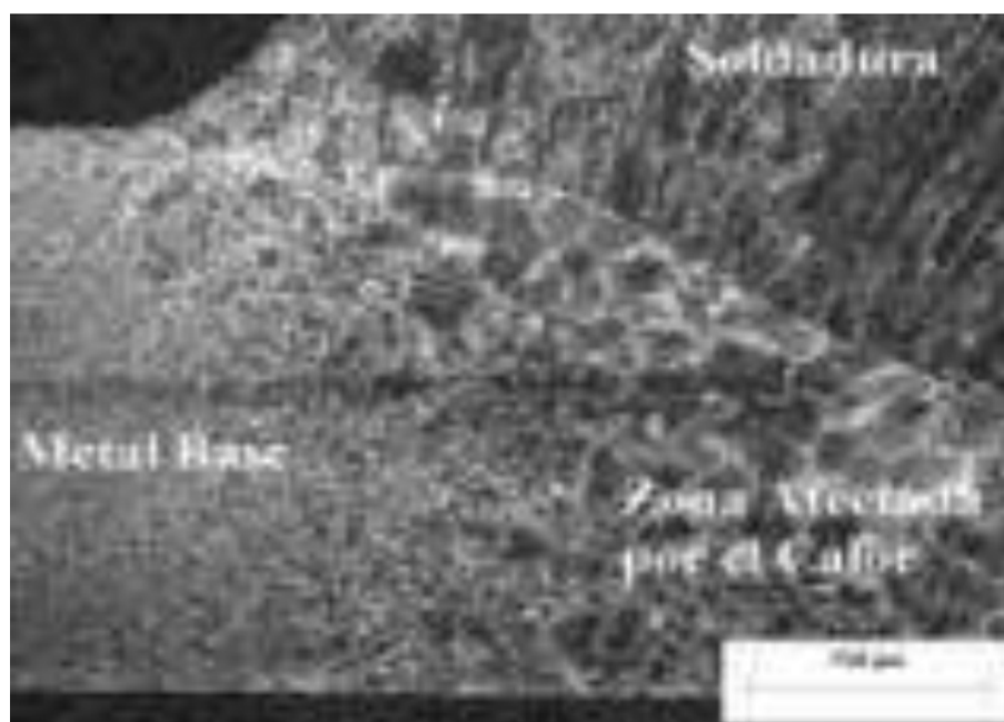
Fig. 5 Microestructura del material soldado
