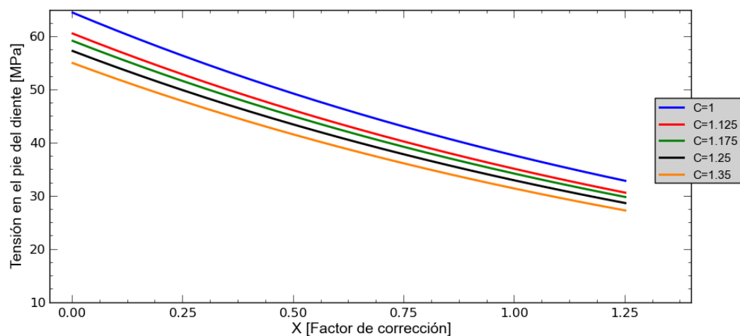
Fig. 6. Variación de las tensiones normales en el eje Z en función de la corrección y del coeficiente de asimetría para un ángulo del perfil del diente en la zona de ataque de 20^\circ
