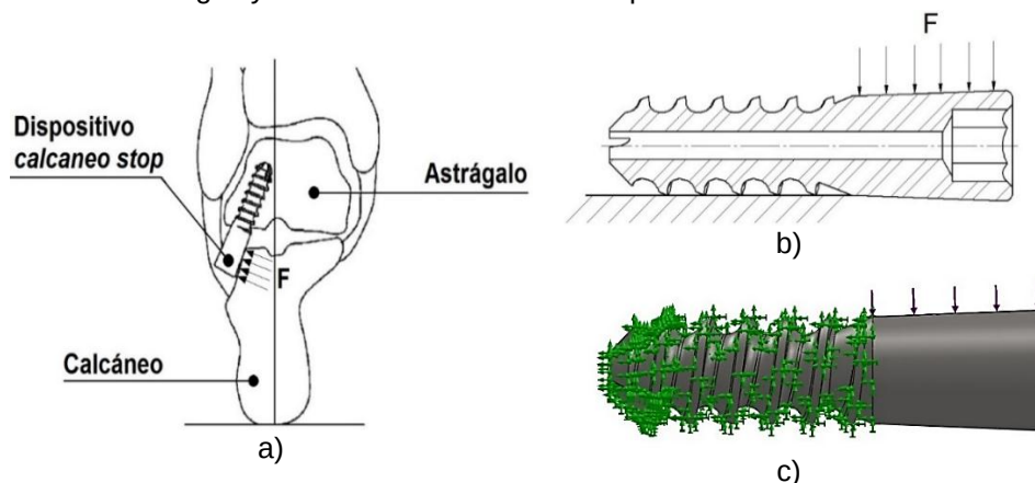
Fig. 3. Modelo de carga del implante calcáneo stop de acuerdo a la colocación en el pie: a) Modo de inserción del implante para lograr la bóveda plantar enroscado en el hueso astrágalo, y la cabeza realiza función de tope, b) representación de las condiciones de cargas, sobre la cabeza se aplica una carga distribuida y un empotramiento en la rosca, c) Representación del modelo de cargas en el software de simulación, las flechas verdes eliminan el movimiento
