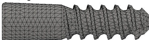
Fig. 4. Mallado del implante calcáneo stop
