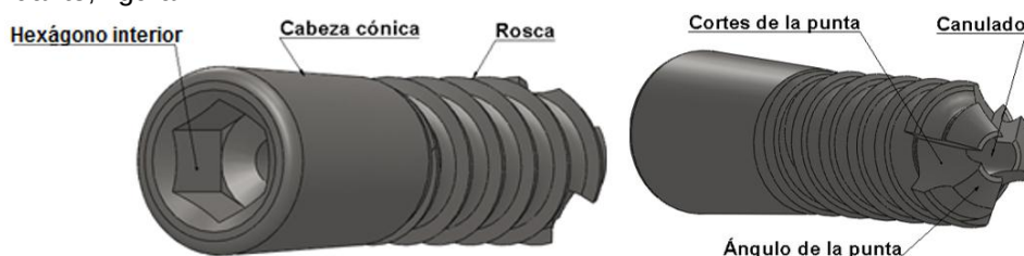
Fig. 1. Modelo geométrico del implante calcáneo stop
