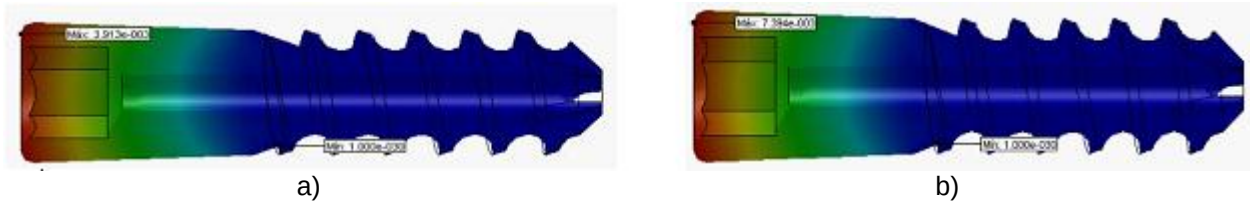
Fig. 7. Gráficos de desplazamientos en el implante calcáneo stop . a) 3,913 \mu\text{m} para el acero inoxidable AISI 316L, b) 7,394 \mu\text{m} para la aleación de Titanio Ti-6Al-4V
