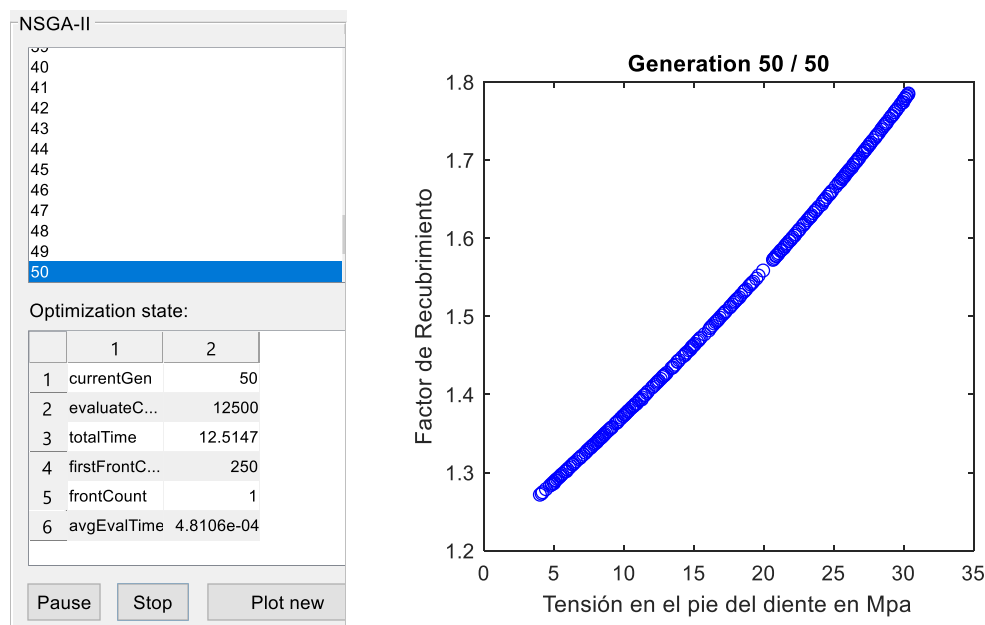
Fig. 4. Frente de Pareto del factor de recubrimiento de la transmisión y tensión en el pie del diente del piñón. Fuente: NSGA II
