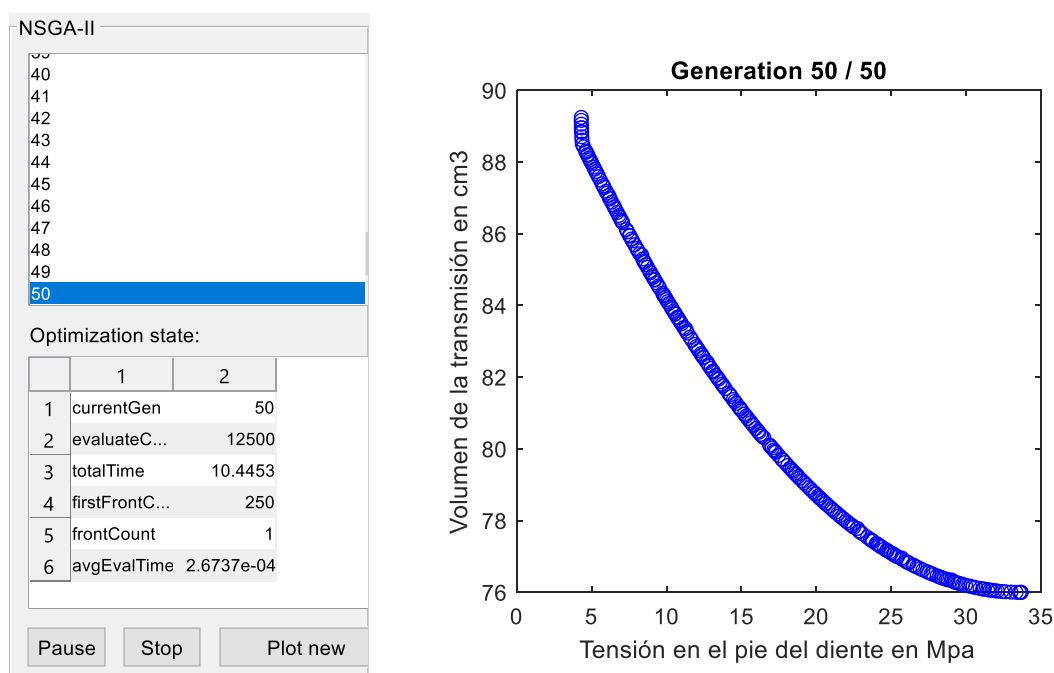
Fig. 5. Frente de Pareto del volumen de la transmisión y tensión en el pie del diente del piñón. Fuente: NSGA II
