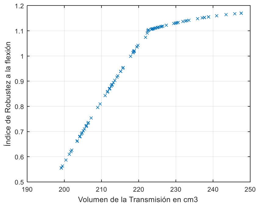
Fig. 3. Frente de Pareto del Índice de Robustez del piñón y volumen de la transmisión. Fuente: PESA II
