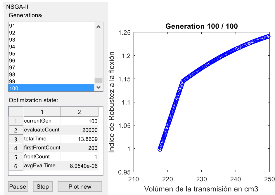
Fig. 2. Frente de Pareto del Índice de Robustez del piñón y volumen de la transmisión. Fuente: NSGA II
