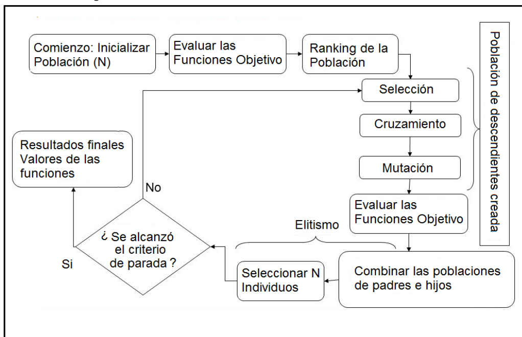
Fig. 1. Diagrama de bloques del algoritmo utilizado NSGA-II. Fuente: adaptada de [14]
