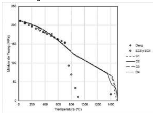
Fig. 7. Valores del módulo de Young en función de la temperatura. b) Resultados estadísticos. Fuente: autores
