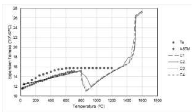
Fig. 6. Comparación de los valores de coeficiente medio de expansión térmica obtenida en función de la temperatura. b) Resultados estadísticos de la comparación. Fuente: autores
