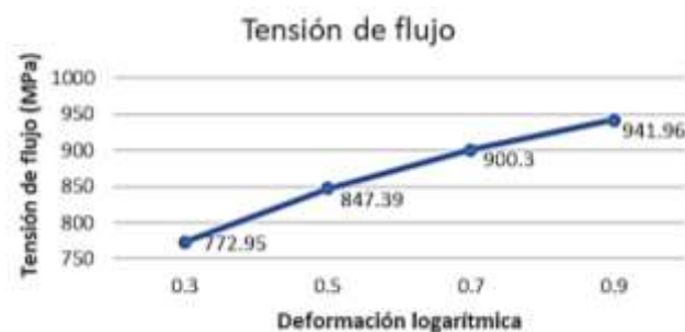
Fig. 5. Gráfico de tensión de flujo respecto a la deformación logarítmica. Fuente: autores
