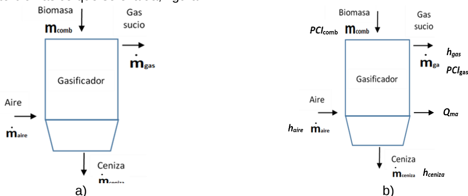
Fig. 2. Esquema del balance de masa a) y de energía b) en el gasificador. Fuente: autores
