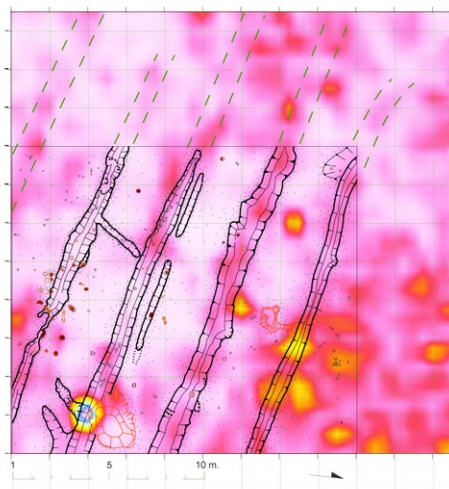
Figura 14. Resultado de las investigaciones con GPR en el Corte F e interpretación, profundidad 60 cm (GPR: Julián Gallego, elaboración A. Sarcina 2015).
