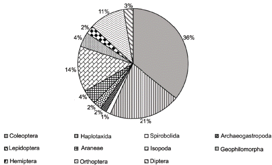
Figura 1. Representación porcentual del número de individuos en el sistema de pastos naturales.
