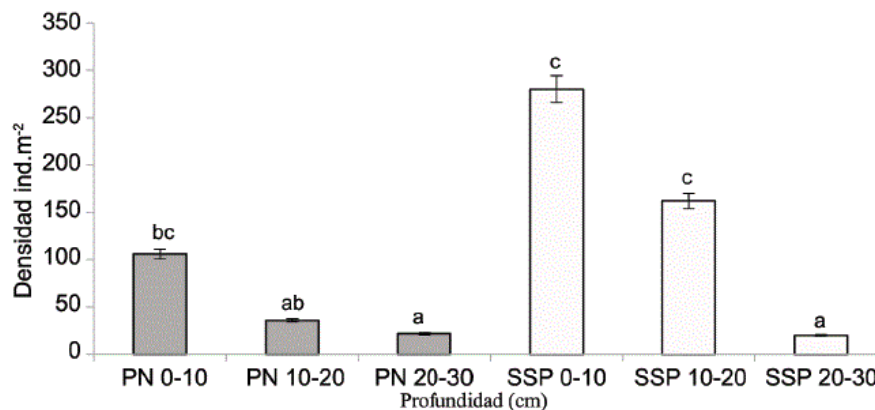
Figura 5. Densidad promedio de la macrofauna del suelo. Período poco lluvioso.
