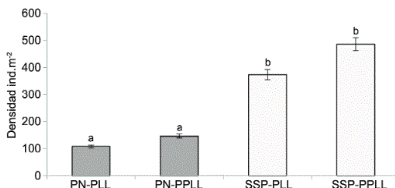
Figura 3. Densidad promedio de la macrofauna en la hojarasca.
