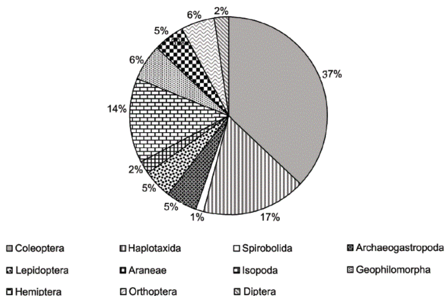
Figura 2. Representación porcentual del número de individuos en el sistema silvopastoril.
