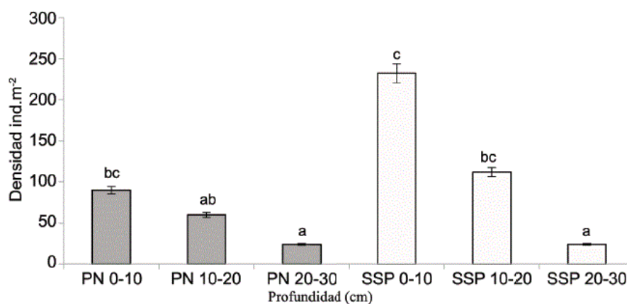
Figura 4. Densidad promedio de la macrofauna del suelo. Período lluvioso.
