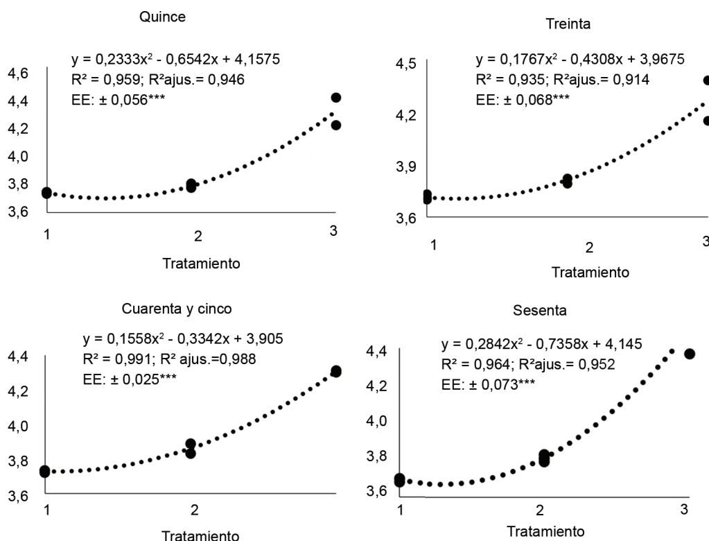
Figura 1. Regresión del pH en el ensilaje y el porcentaje de forraje de M. esculenta , variedad INIVIT Y-93-4, en correspondencia con los momentos de muestreo.
