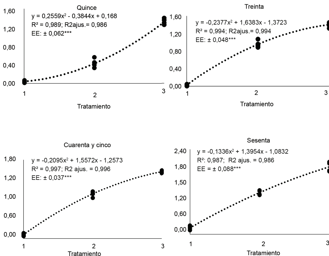
Figura 3. Regresión del N-NH 3 en el ensilaje y el porcentaje de forraje de M. esculenta , variedad Señorita, en correspondencias con los momentos de muestreo.
