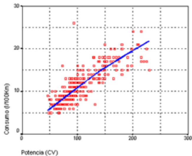
Figura 1. Correlación entre potencia y consumo de motor.
