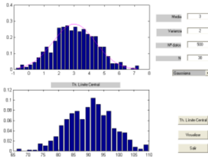
Figura 4. Submenú variable aleatorias.
