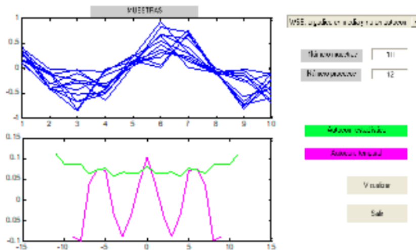
Figura 5. Autocorrelación.
