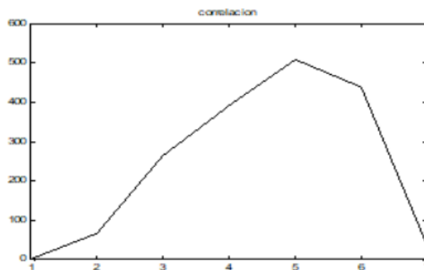
Figura 6. Correlación.
