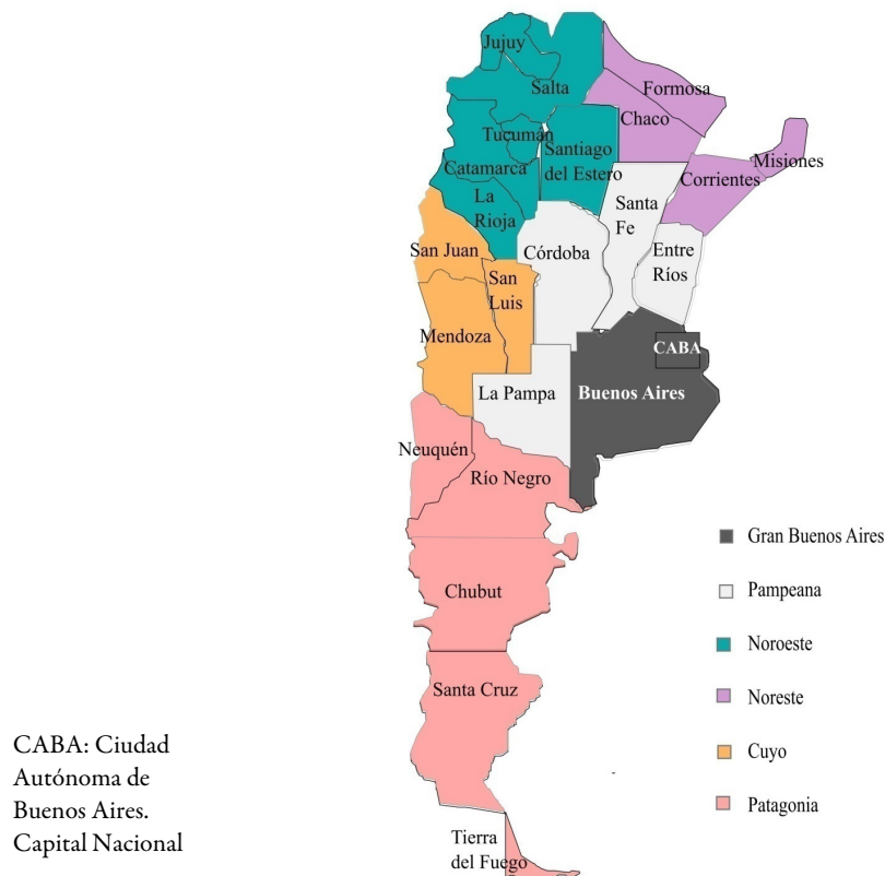
FIGURA A1. Mapa de las provincias argentinas
