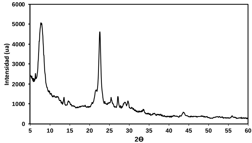
Figura 2. Difractograma de la zeolita beta ( Z\beta ).
