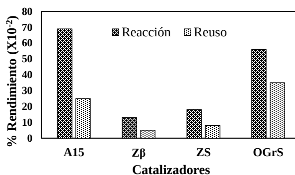
Figura 12. Porcentaje de rendimiento con un reúso del catalizador A15.
