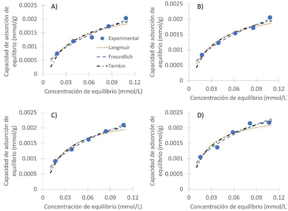
Figura 7. Representación de los modelos de isothermas ajustados a las temperaturas a. 25 °C, b. 30 °C, c. 35 °C y d. 40 °C para la remoción de azul brillante en cáscara de yuca modificada con ácido fosfórico. Dosis de biomasa: 10 g/L, Temperatura: 25°C, pH: 2.1. Fuente: propia
