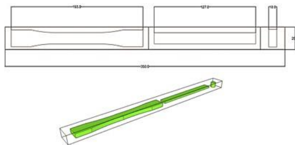
Figura 4. Distribución geométrica de las probetas en las barras de compuesto extrudidas.
