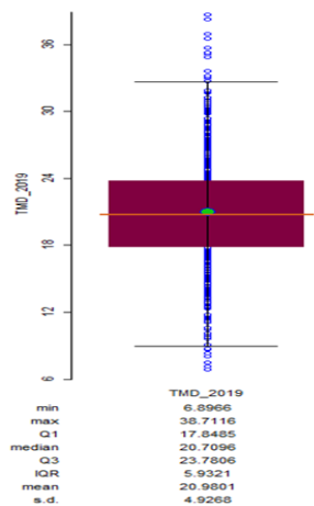
Figura 1: Diagrama de caja TMD 2019.
