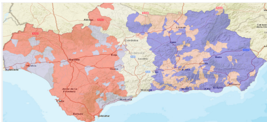
Mapa 2: LISA PROYECTADO MATRIZ D3_36Km.
