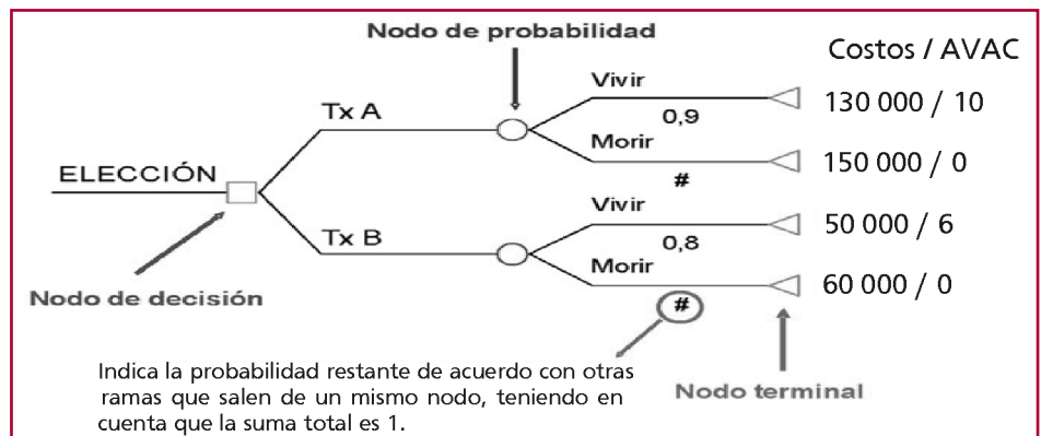
Fig. 3. Ejemplo de árbol de decisión de Markov.
