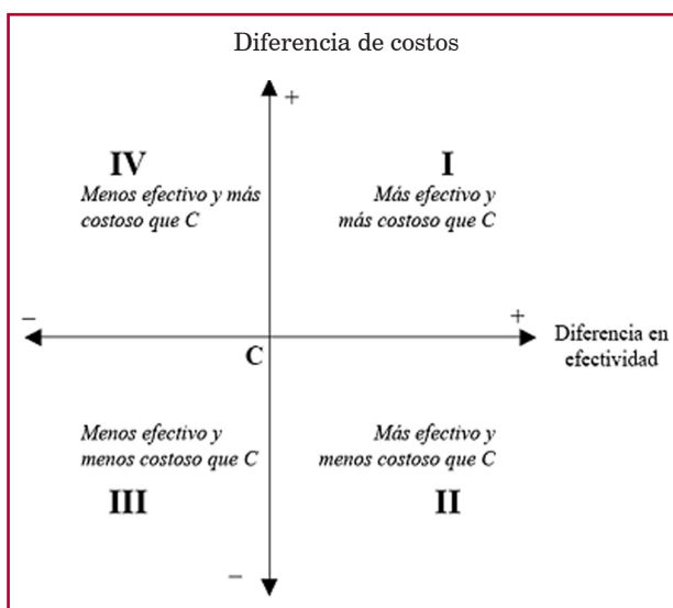
Fig. 1. Análisis Costo-efectividad. Posición II. Más efectivo y menos costoso.
