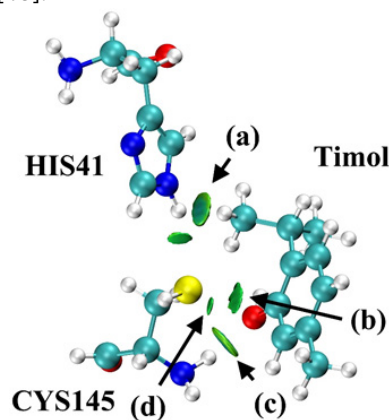
Figura 13. Isosuperficie IGMH para la interacción entre el timol y los residuos HIS41 y CYS145 de la proteasa 3CLpro.
